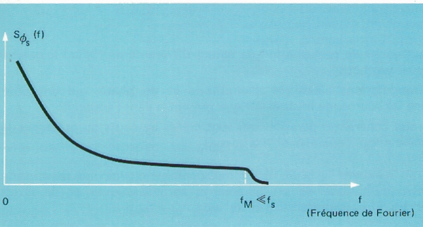
Fig. 1 allure de S_{\phi_s}(f)
