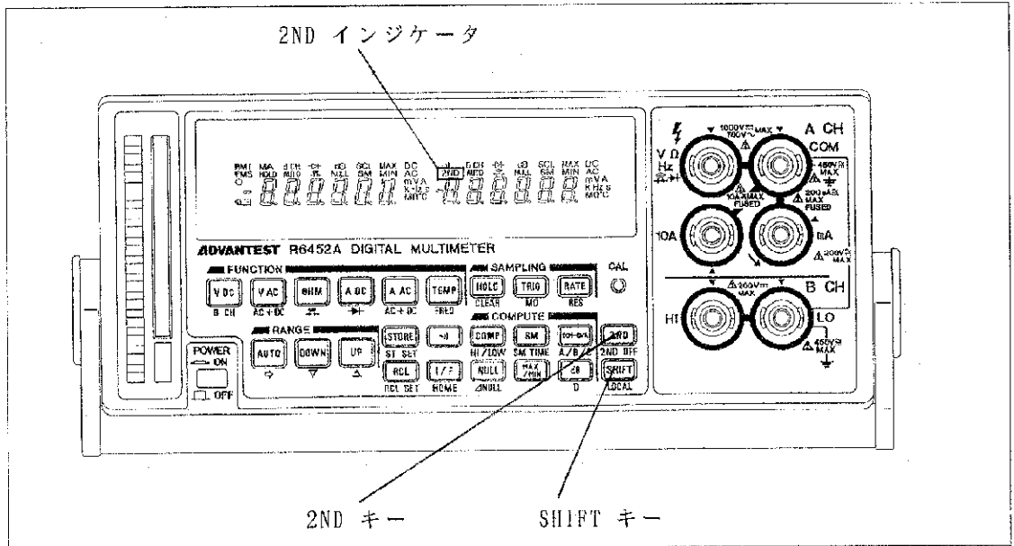
図 5 - 4 第2 表示に関わるキー
