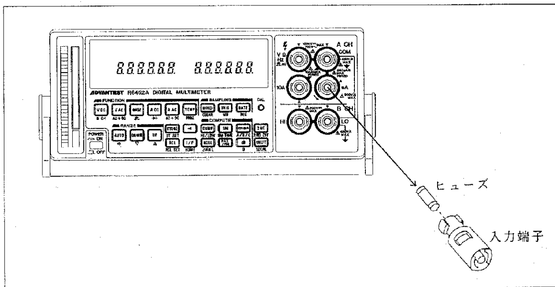
図 2 - 4 mA入力端子保護用ヒューズ
