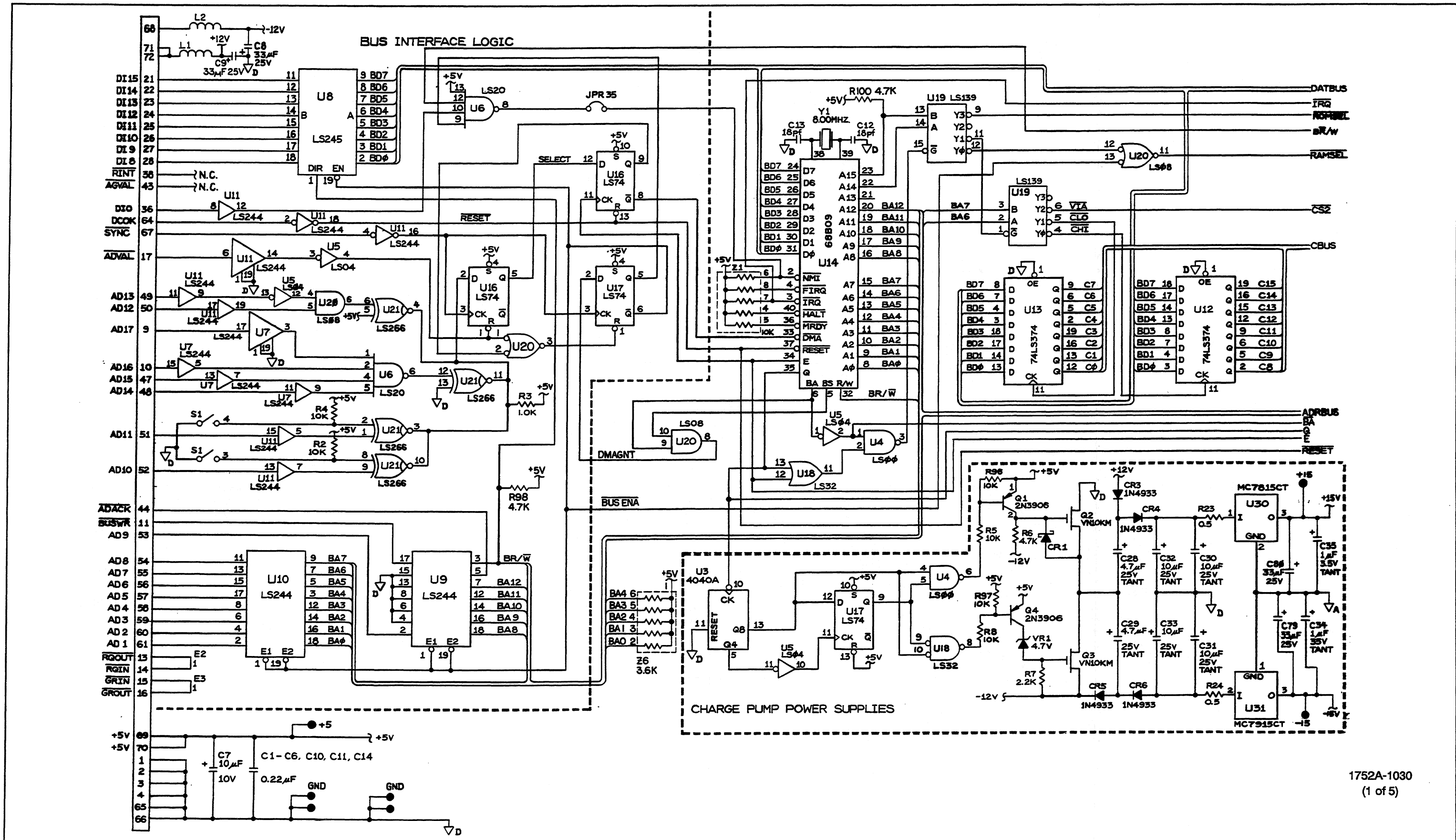
Figure 5-11. 010 A/D Converter Module (cont)
