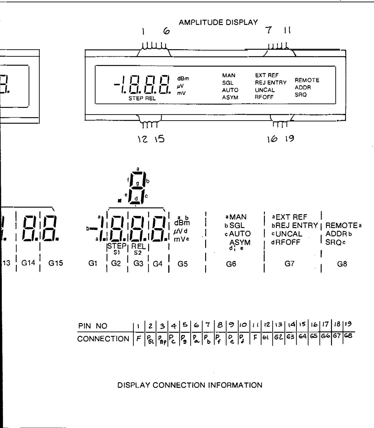
Figure 8-5. A1A1 Display PCA (cont)
