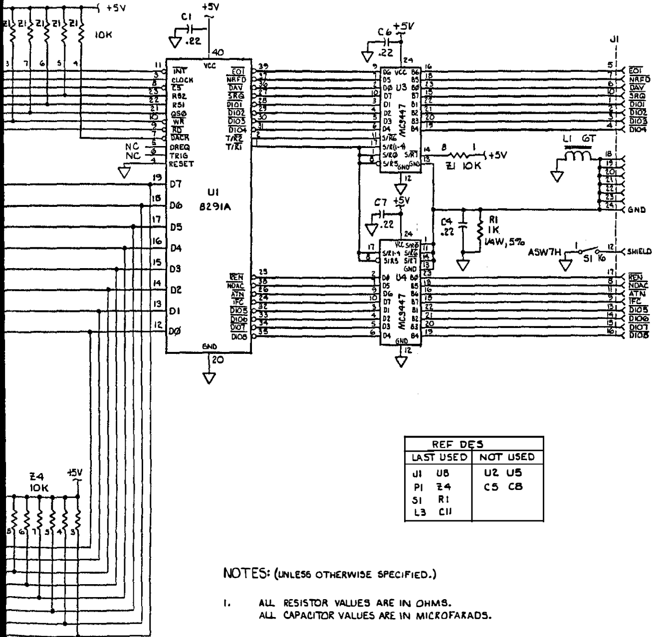
Figure 8-16. A3A3A1 IEEE-488 Interface PCA (Option -488)
