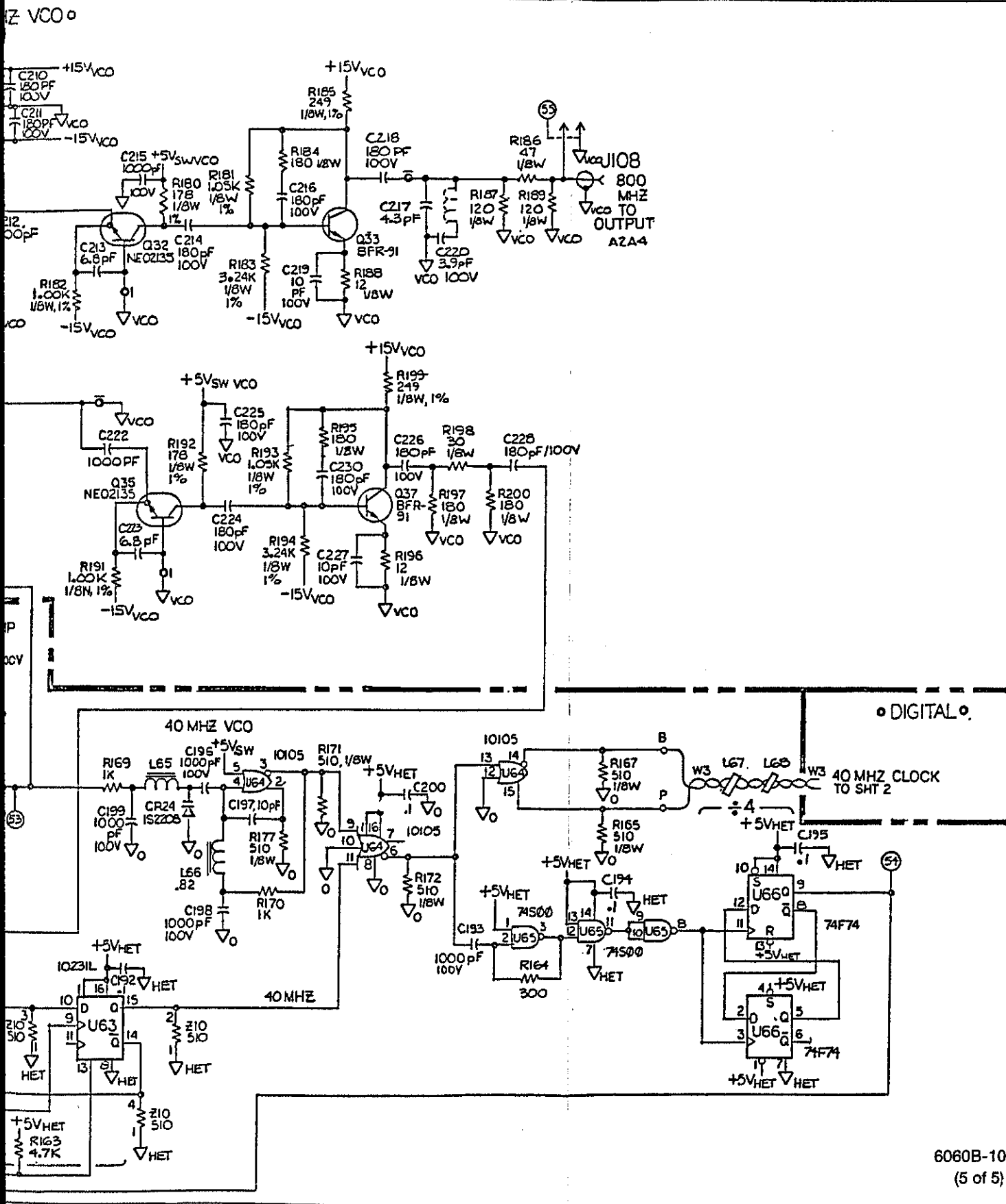
Figure 8-6. A2A1 Synthesizer PCA (cont)
