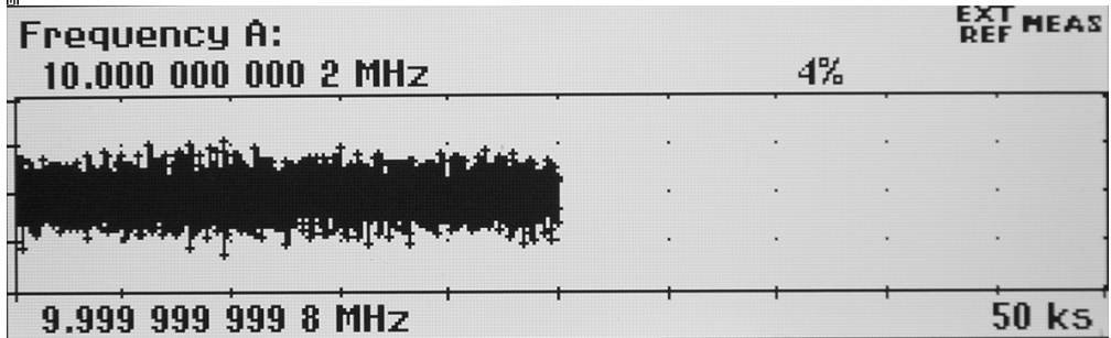
HP Z3805 ExRef und DUT Plot 5SekGt SmartFrequ on 7 h verlauf.JPG (198.03 kB, 1180x357 - viewed 196 times.)
