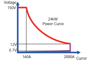
PEL-5024C-150-2000
