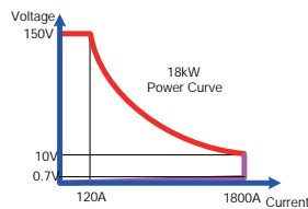
PEL-5018C-150-1800
