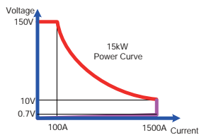
PEL-5015C-150-1500
