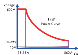
PEL-5008C-600-560
