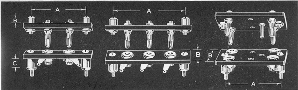
TYPE 274-CP TYPE 274-CJ
