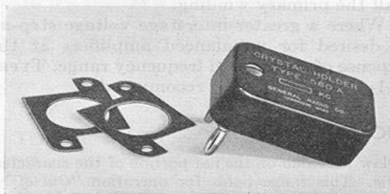
TYPE 560-A Crystal Holder
