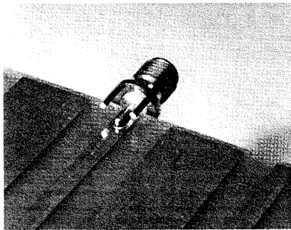
Figure 19. SMA Edge Launcher
