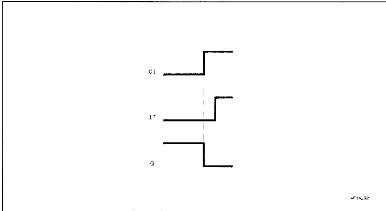
Figure 7D-3. IT Lagging CI
