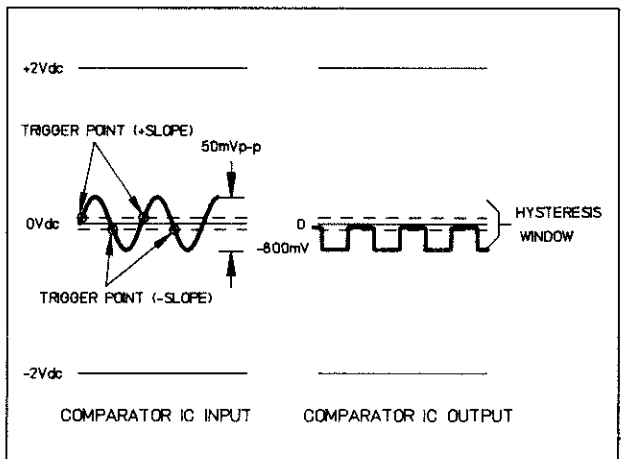
(D) +1 VDC OFFSET
