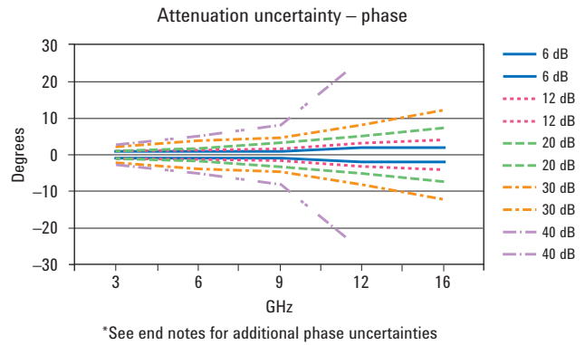
Attenuation
