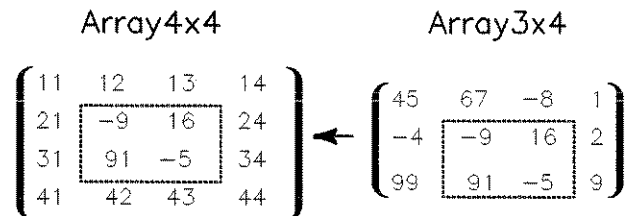
Copying a Subarray into Another Subarray
