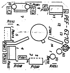
PEF-6270D PCB
