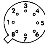
TO-99
