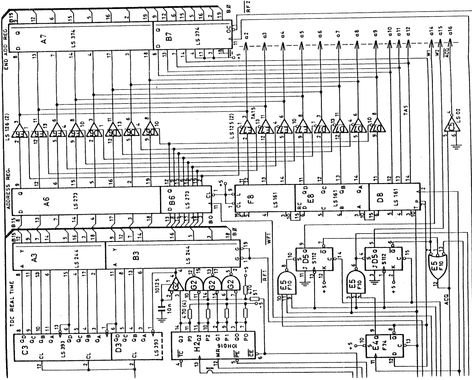
LeCroy 9400-4-S1 Sheet 5 of 7 Eco:1011
