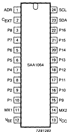
Fig. 2 Pinning diagram.
