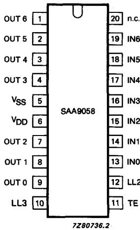
Fig. 2 Pinning diagram.
