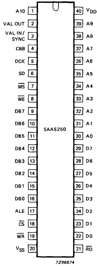
Fig. 2 Pinning diagram.
