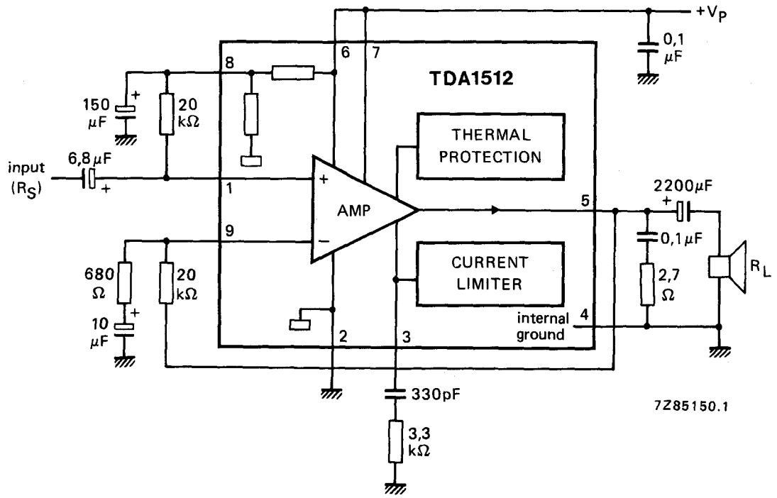
Fig. 3 Test circuit.
