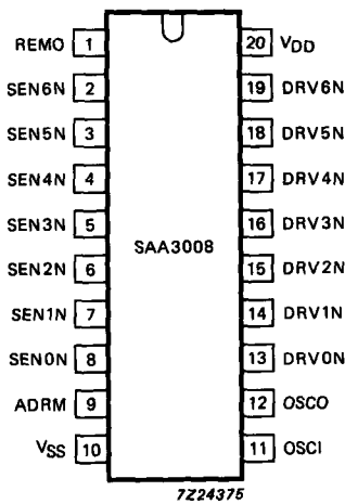
Fig.2 Pinning diagram.
