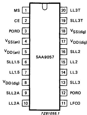
Fig. 2 Pinning diagram.
