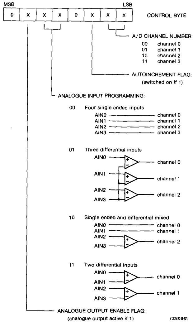
Fig. 4 Control byte.
