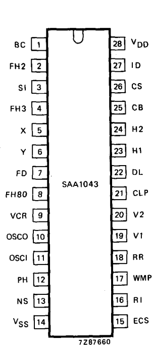
Fig. 2 Pinning diagram.
