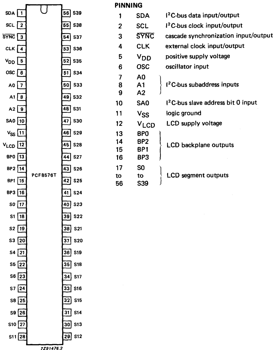
Fig. 2 Pinning diagram.
