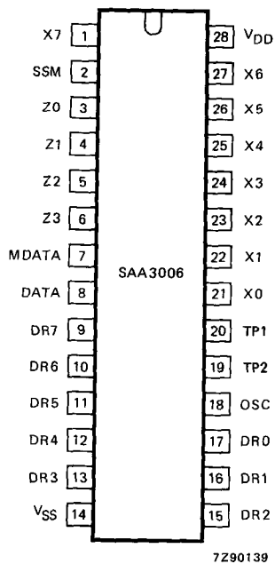
Fig. 2 Pinning diagram.
