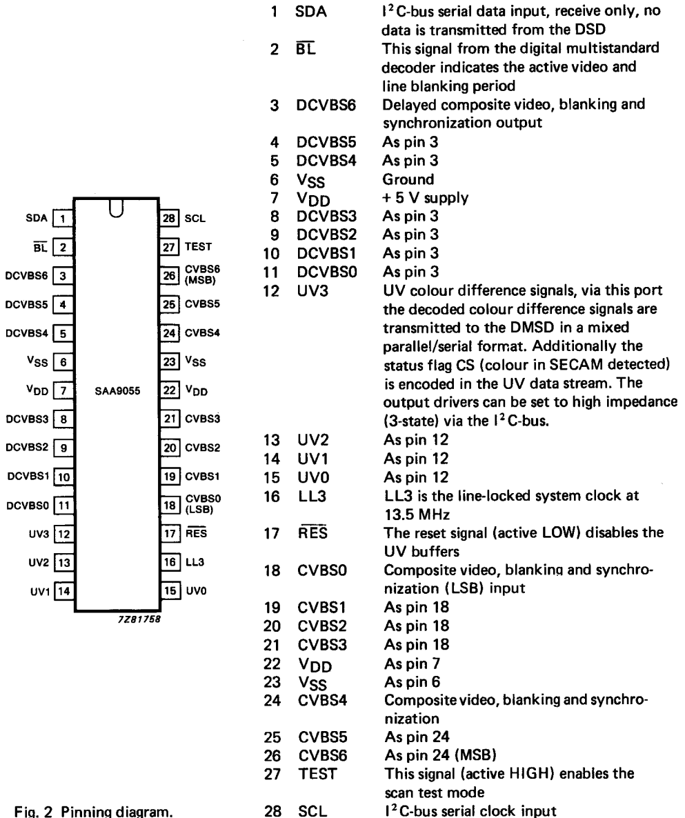
Fig. 2 Pinning diagram.
