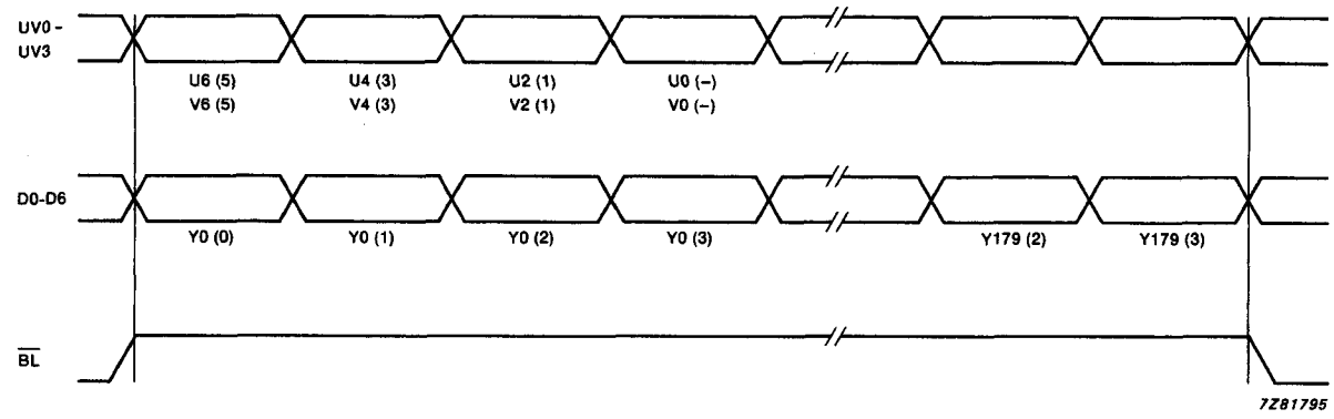
Fig.3 Data format.
