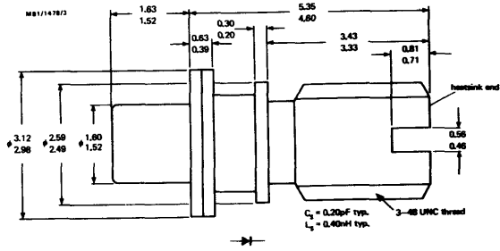
case style MO-66
