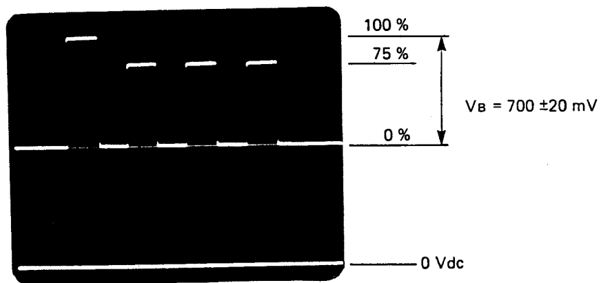
Fig. 36 Output 'BLUE'
