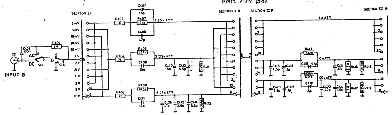
AMPL./DIV. (S8)
