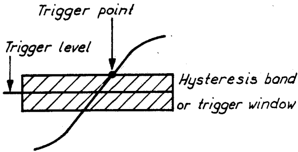
Fig. VI-2. Triggering
