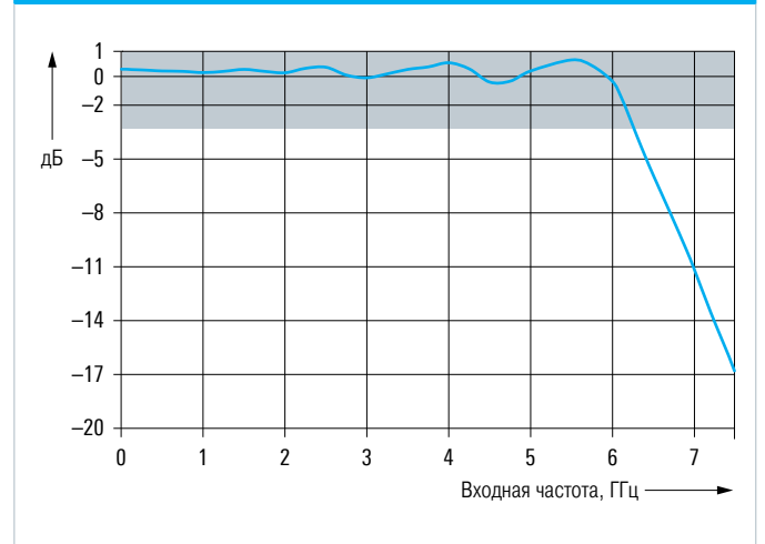
Измеренная АЧХ осциллографа R&S®RTO2064
