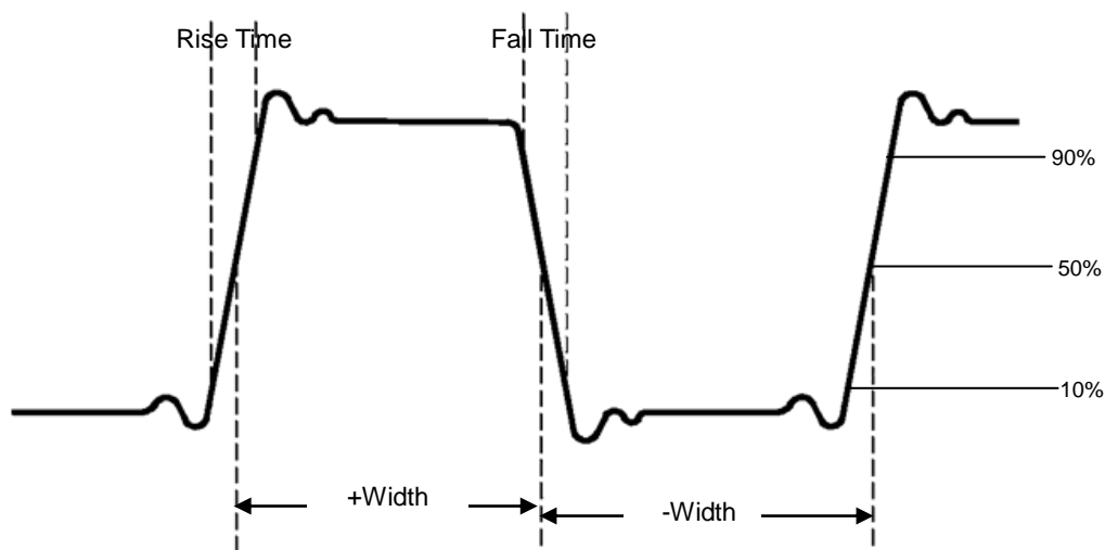
Figure 2- 119 Time parameters
