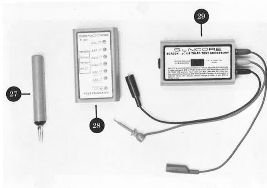
Fig. 4— Optional accessories
