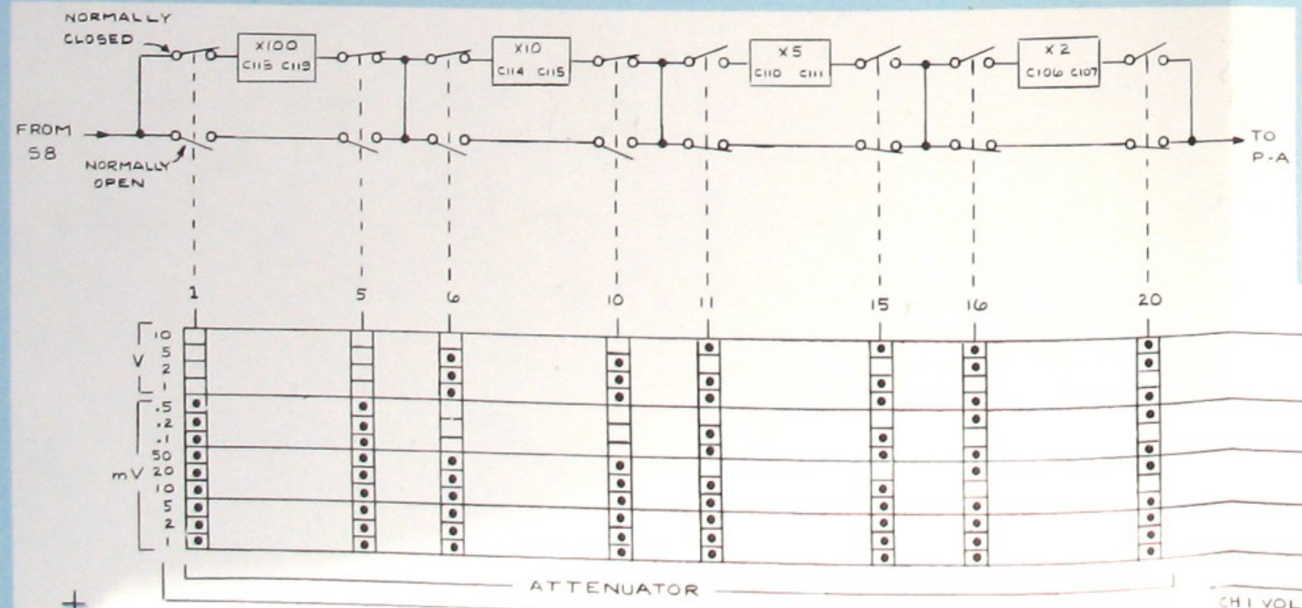
P/O A4 CHI CAM SWITCH
