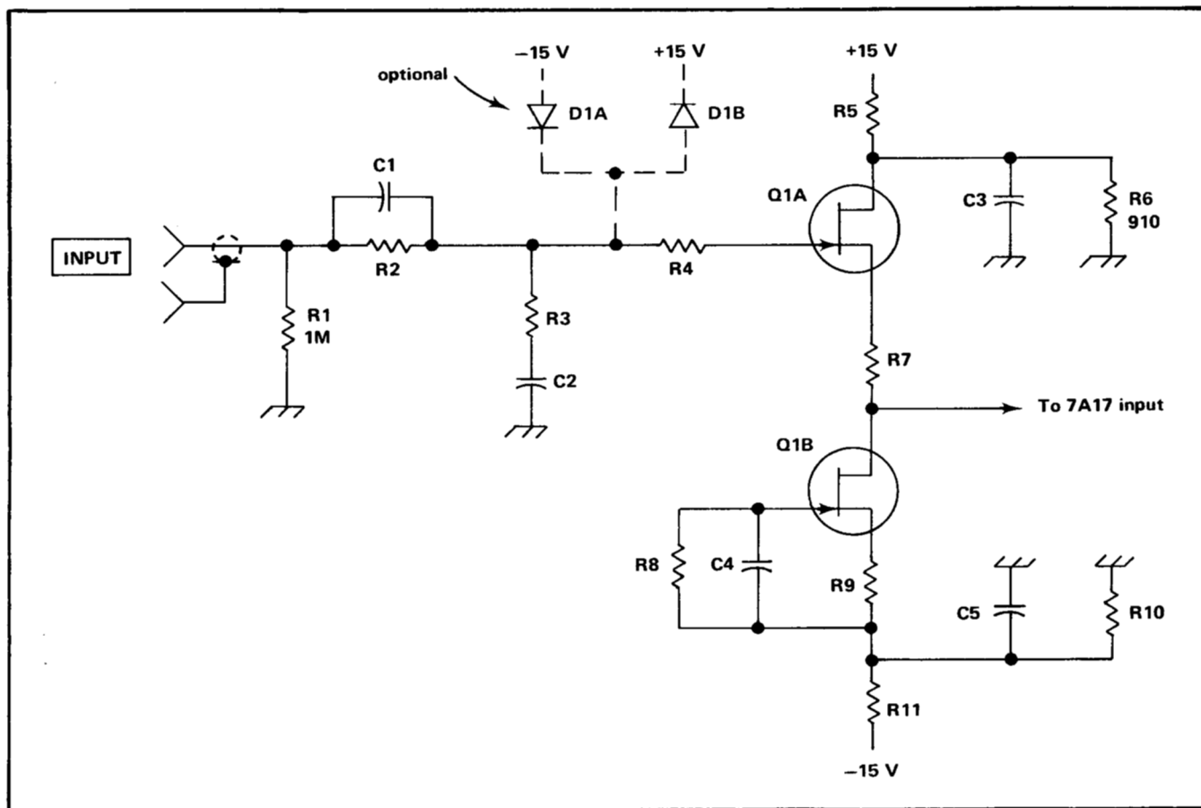
Fig. 3. FET Amplifier.
