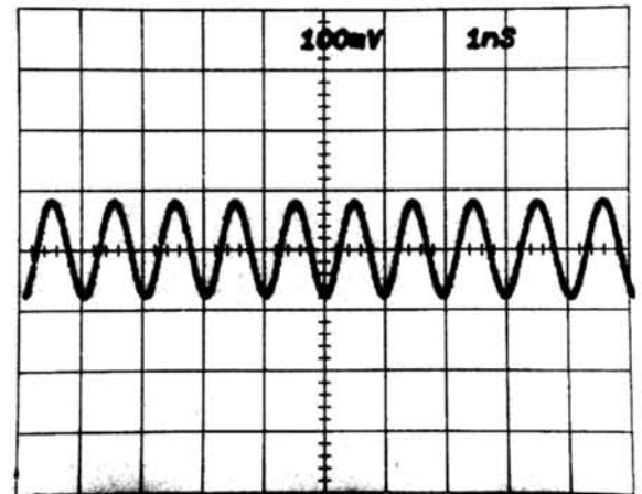
Fig. 7-4. 1 GHz SYNC.
