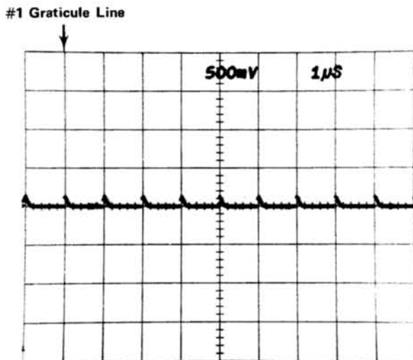
Fig. 7-5. 1 \mu s/DIV.
