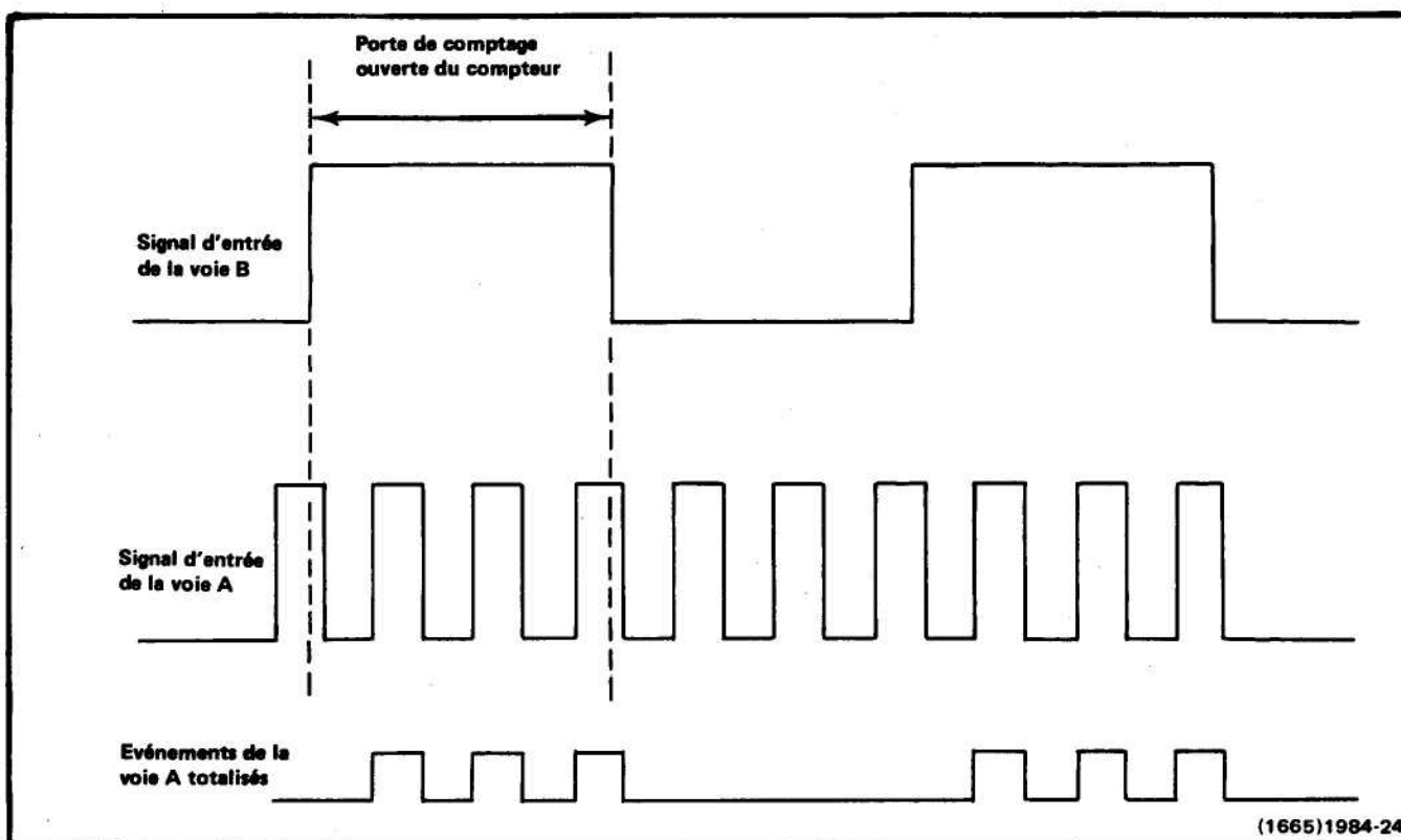
Fig. 2-6. Événements de la voie A comptés à partir d'une fraction d'impulsions de la voie A durant l'ouverture de la porte de comptage (contrôlée par le signal de la voie B).
