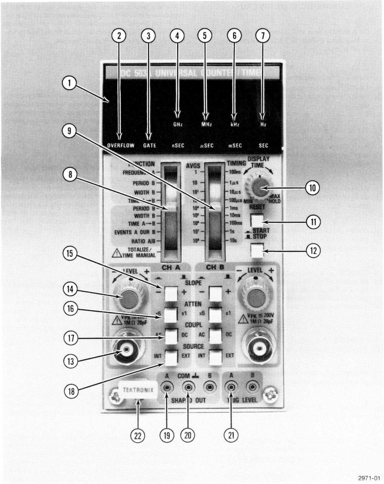
Fig. 2-2. Commandes et prises.
