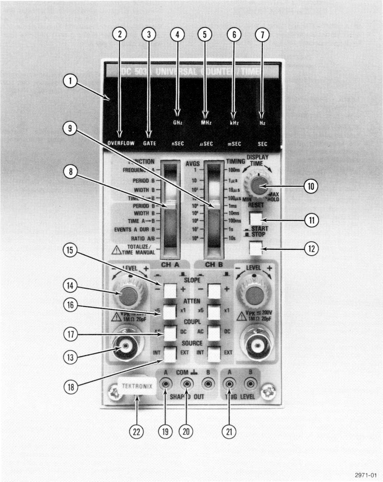
Abb. 2-2: Bedienelemente und Anschlüsse
