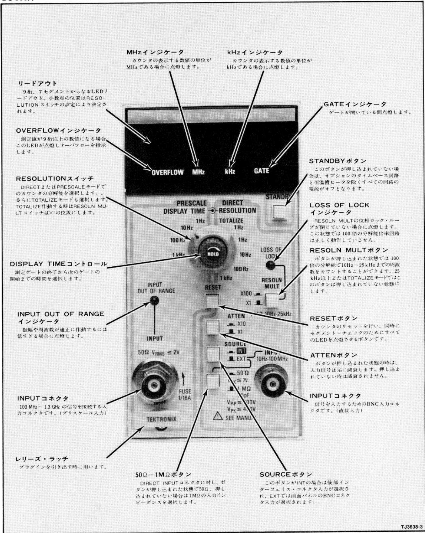
Fig. 2-2. DC 508A コントロールとコネクタ
