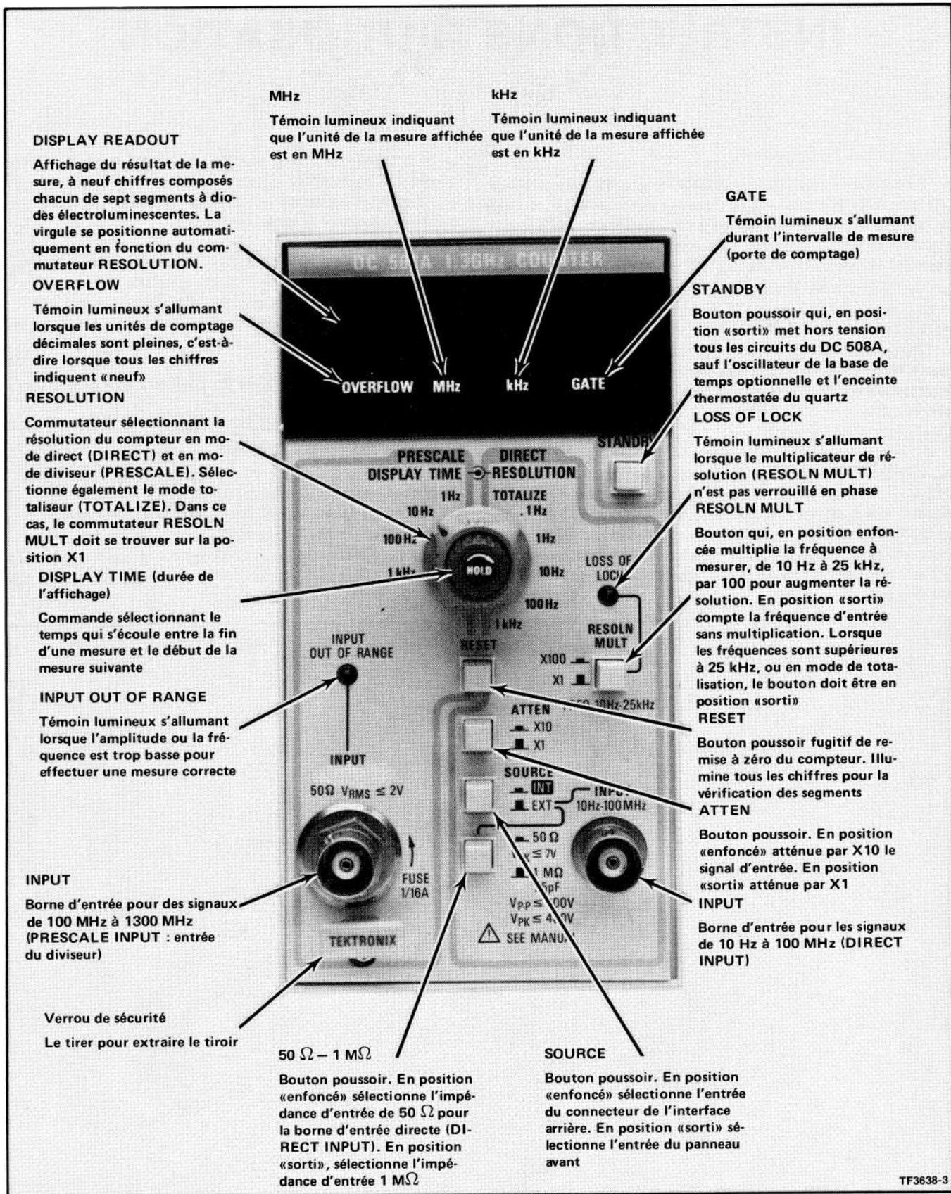
Fig. 2-2. Commandes et prises du DC 508A.
