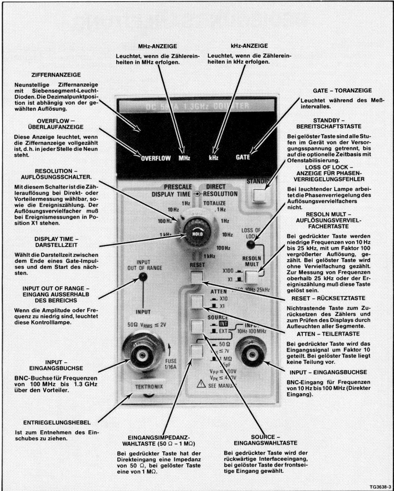
Abb 2-2. Bedienungselemente und Verbindungsbuchsen am DC 508A.
