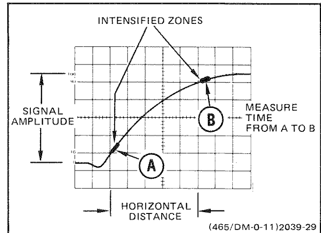
Fig. 32. Risetime.
