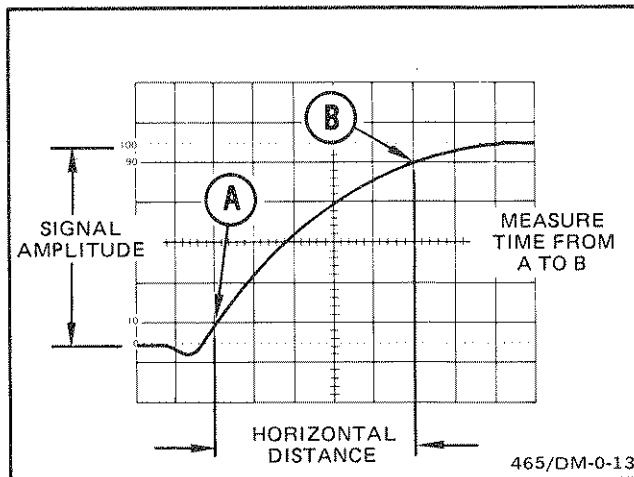
Fig. 19. Risetime.
