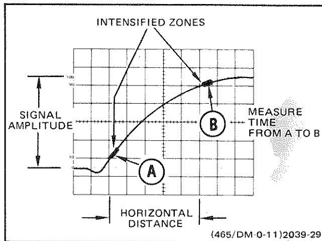
Fig. 32. Risetime.
