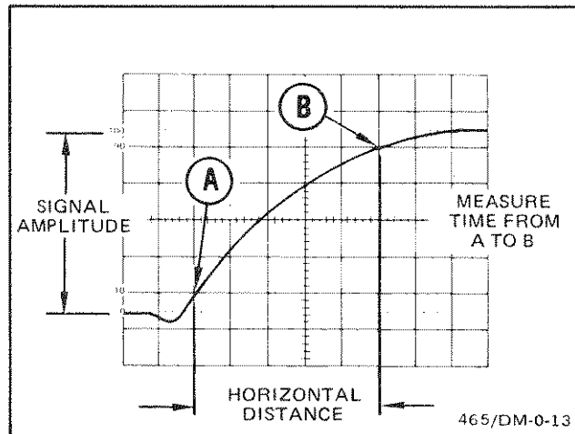
Fig. 19. Risetime.
