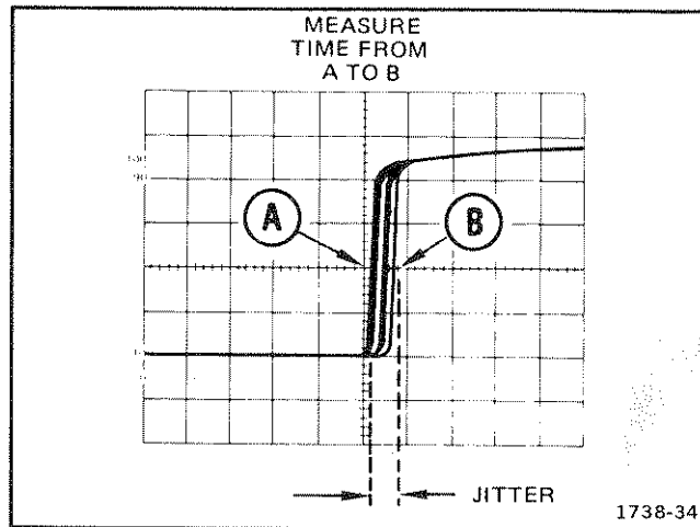
Fig. 23. Pulse jitter.
