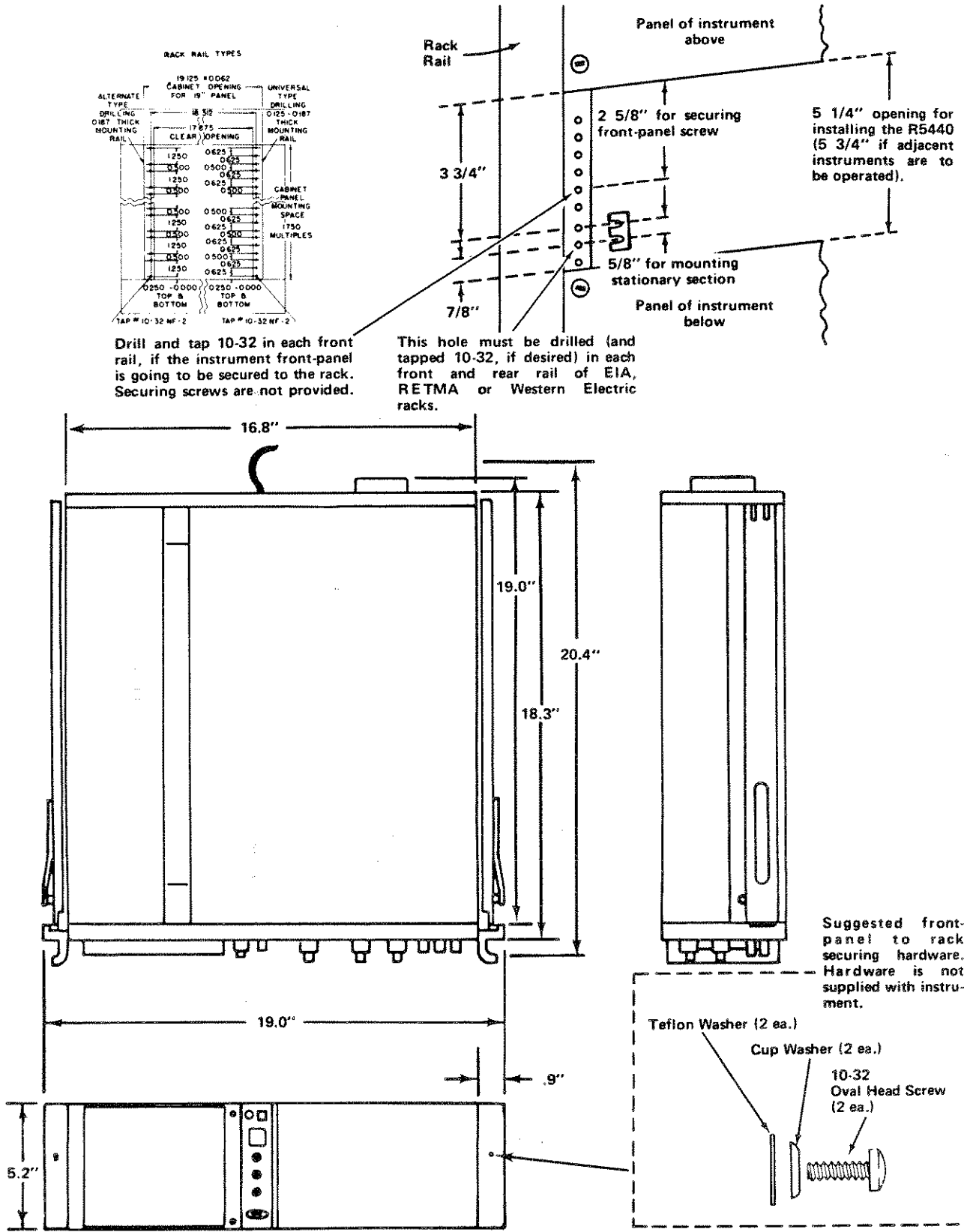
Fig. 1-5. Dimensional diagram.
