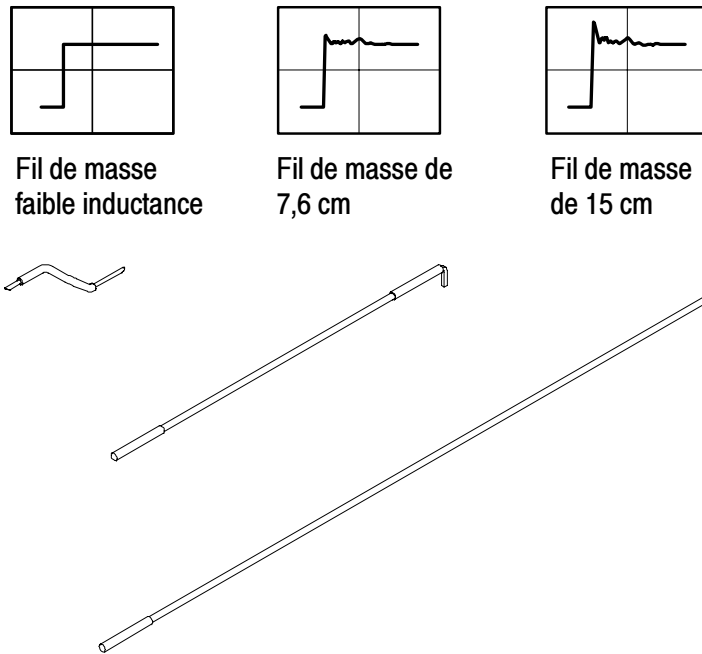
Figure 2-1: Distortion du signal selon la longueur du fil de masse
