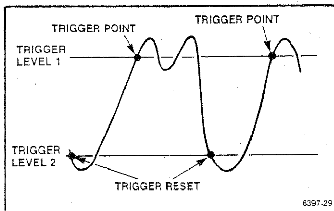
Fig. 3-16. +Hysteresis (Level 1 > Level 2).
