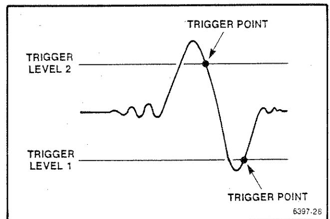
Fig. 3-15. BI slope trigger (Level 2 > Level 1).
