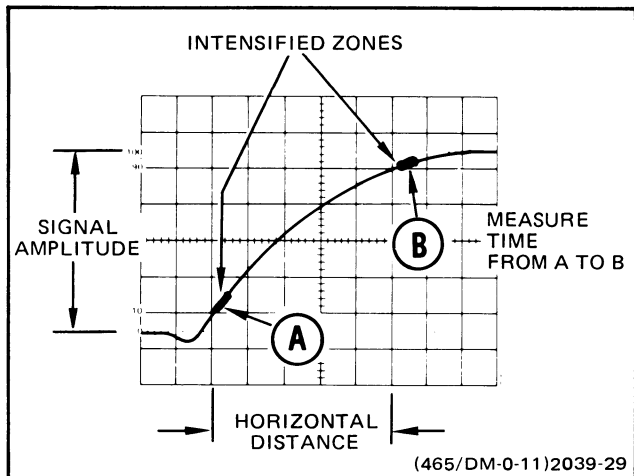
Fig. 28. Risetime.
