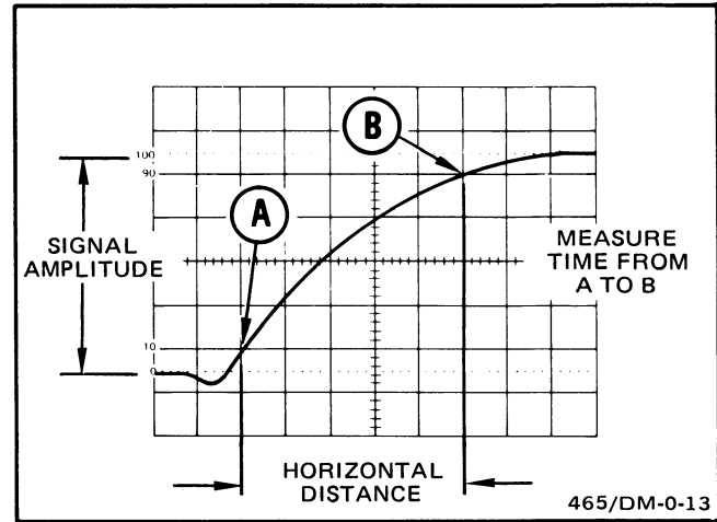
Fig. 19. Risetime.
