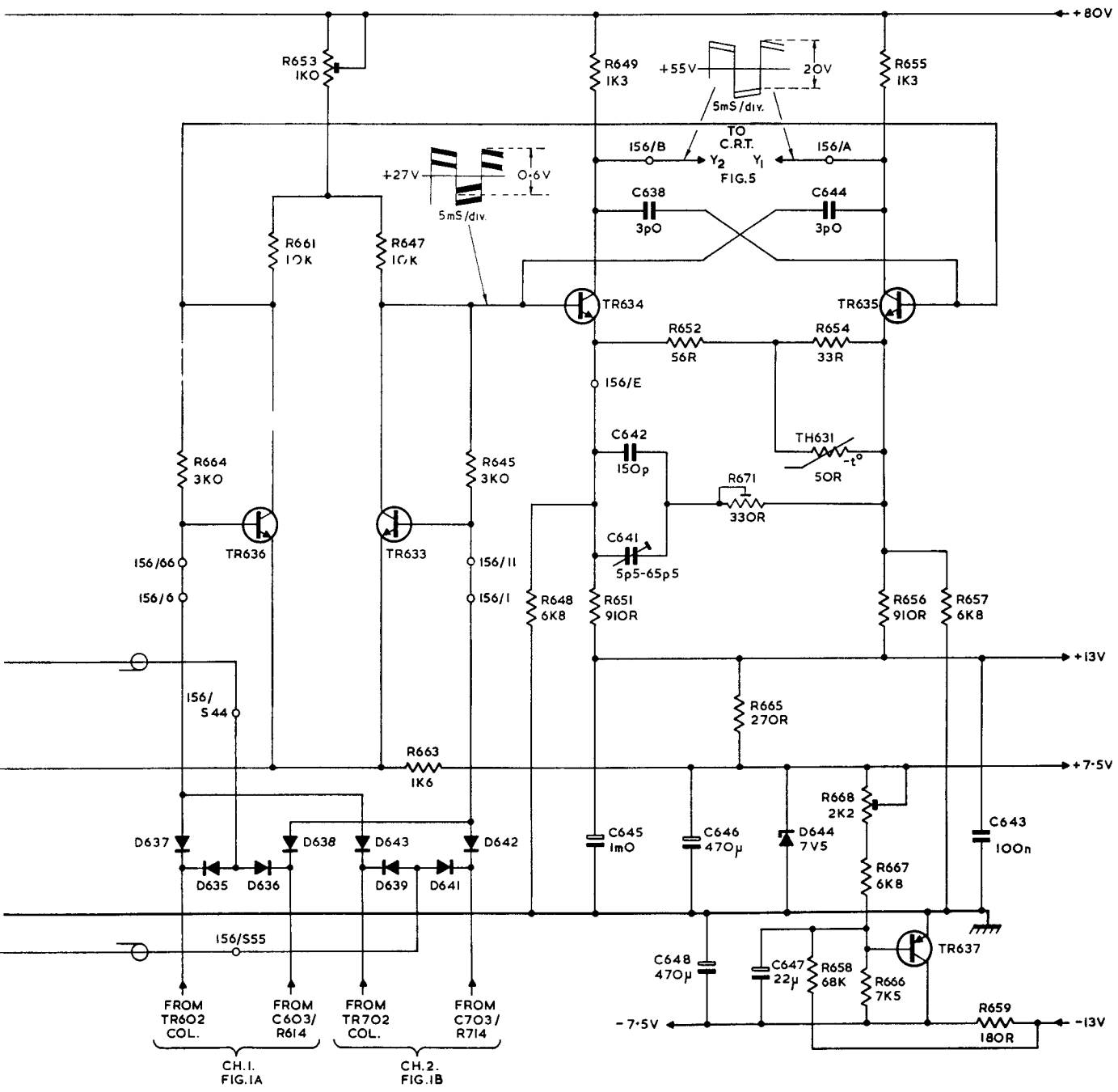
'Y' AMPLIFIER - D61 FIG. 2.
