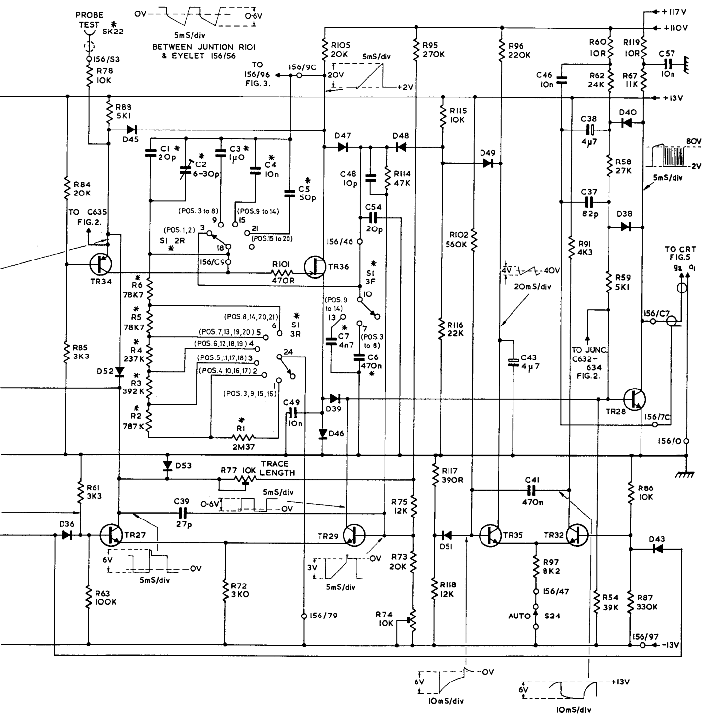
SWEEP GENERATOR D61 FIG. 4.
