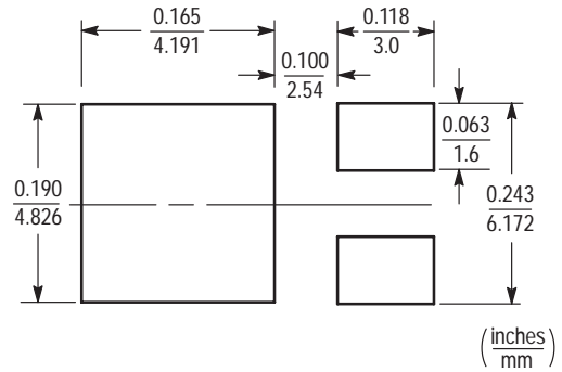
DPAK
