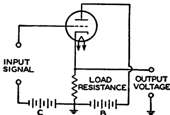
Fig. 51—Cathode-follower circuit.
