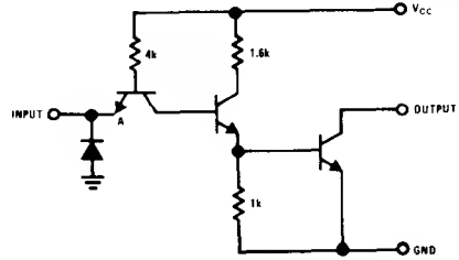
DS7812/DS8812
