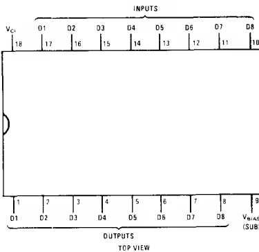
DS8887, DS7897/DS8897
