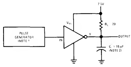
DS8863
