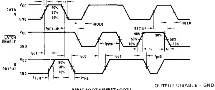
MM54C374/MM74C374
