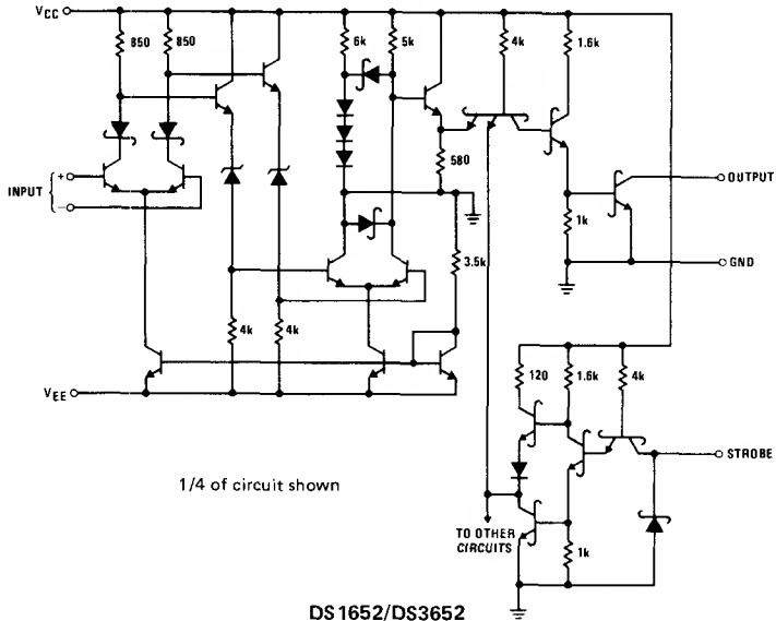
DS1652/DS3652
