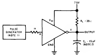
DS75492
