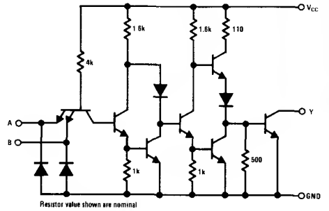
DS55464/DS75464
