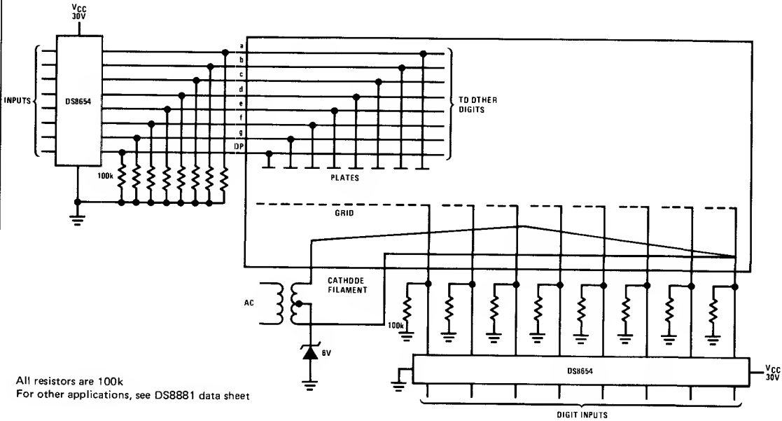
VF Display
