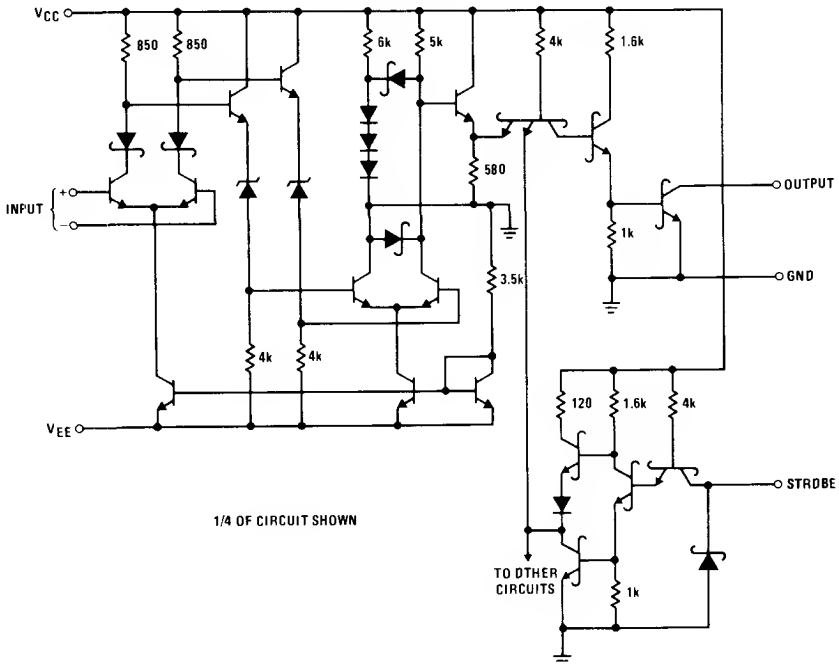
DS1653/DS3653
