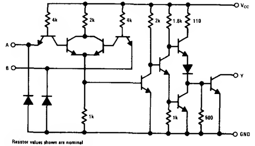
DS55464/DS75464
