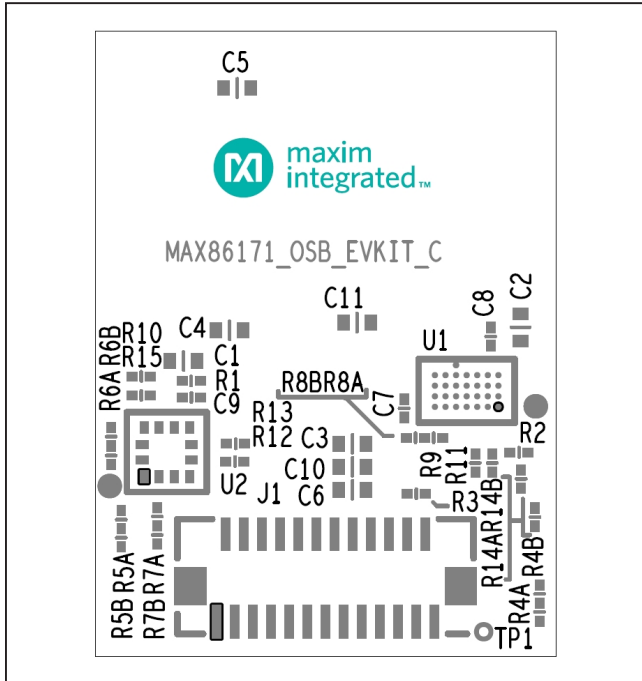
MAX86171OSBEK#—Top Silkscreen
