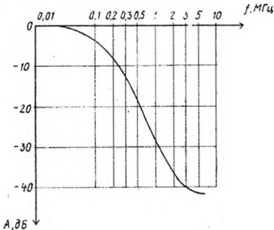
Рис. 3. Кривая зависимости ослабления A фильтра ФНЧ от частоты.
