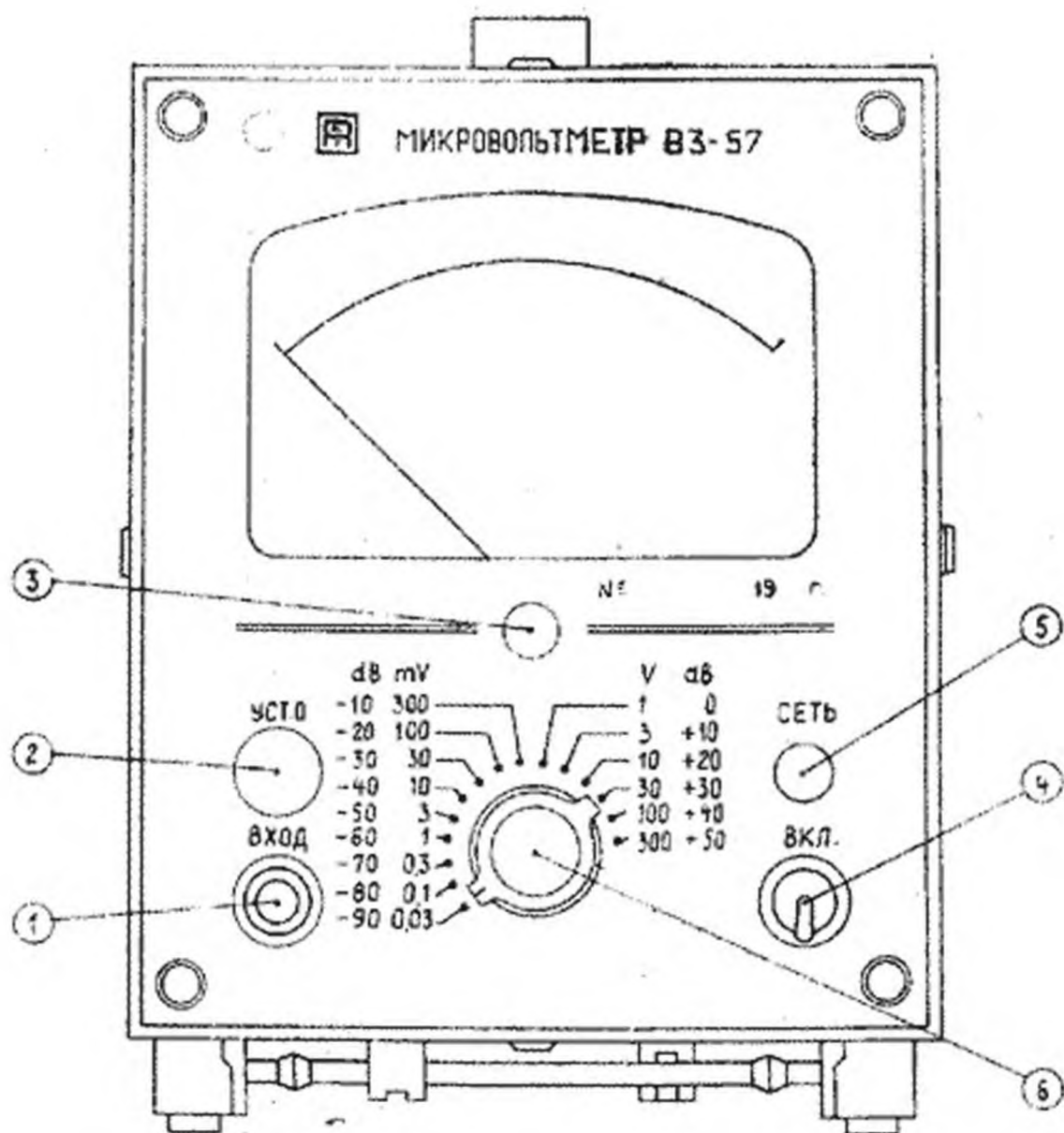
Рис. 4. Вид прибора со стороны передней панели:
