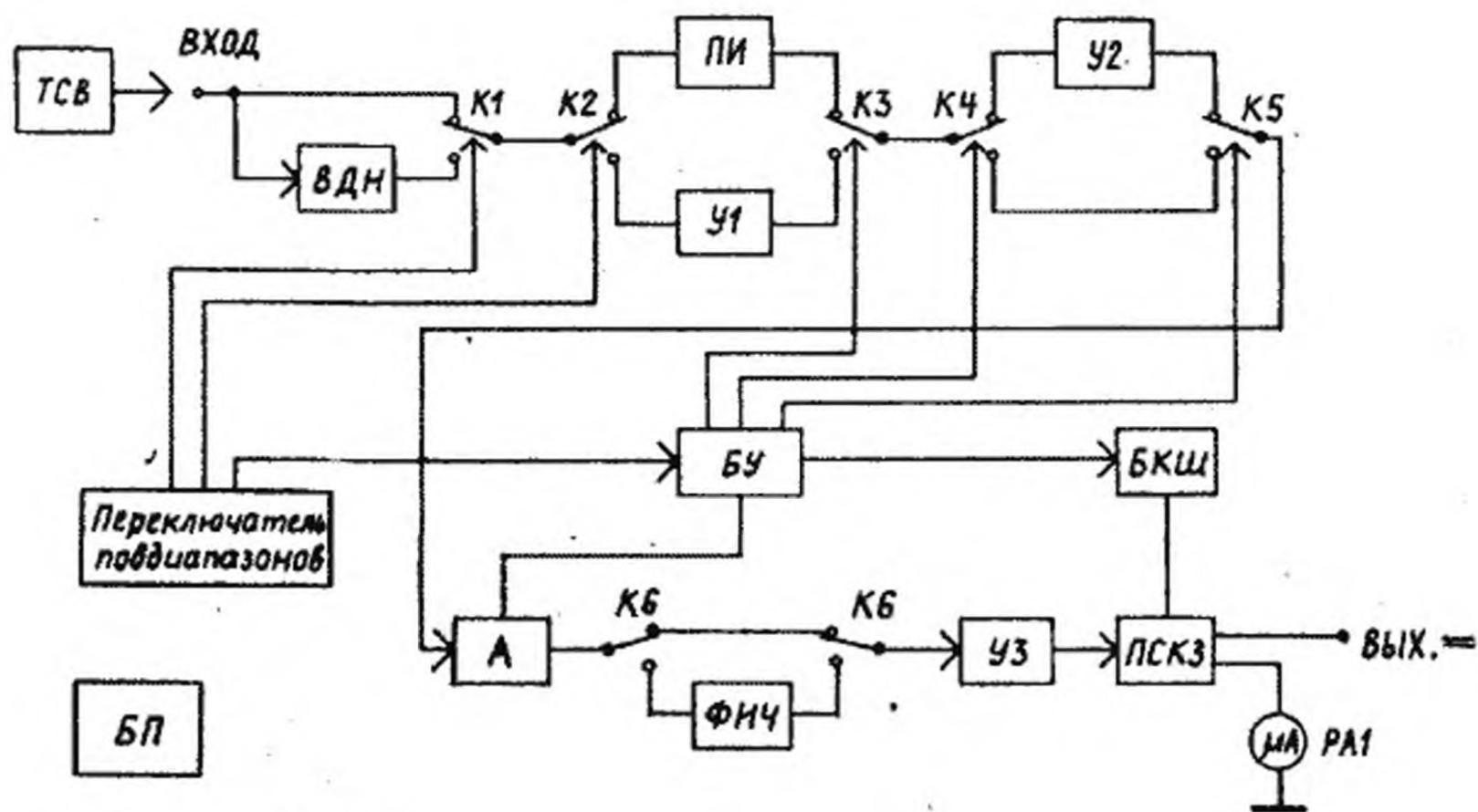
Рис. 2. Схема электрическая структурная
