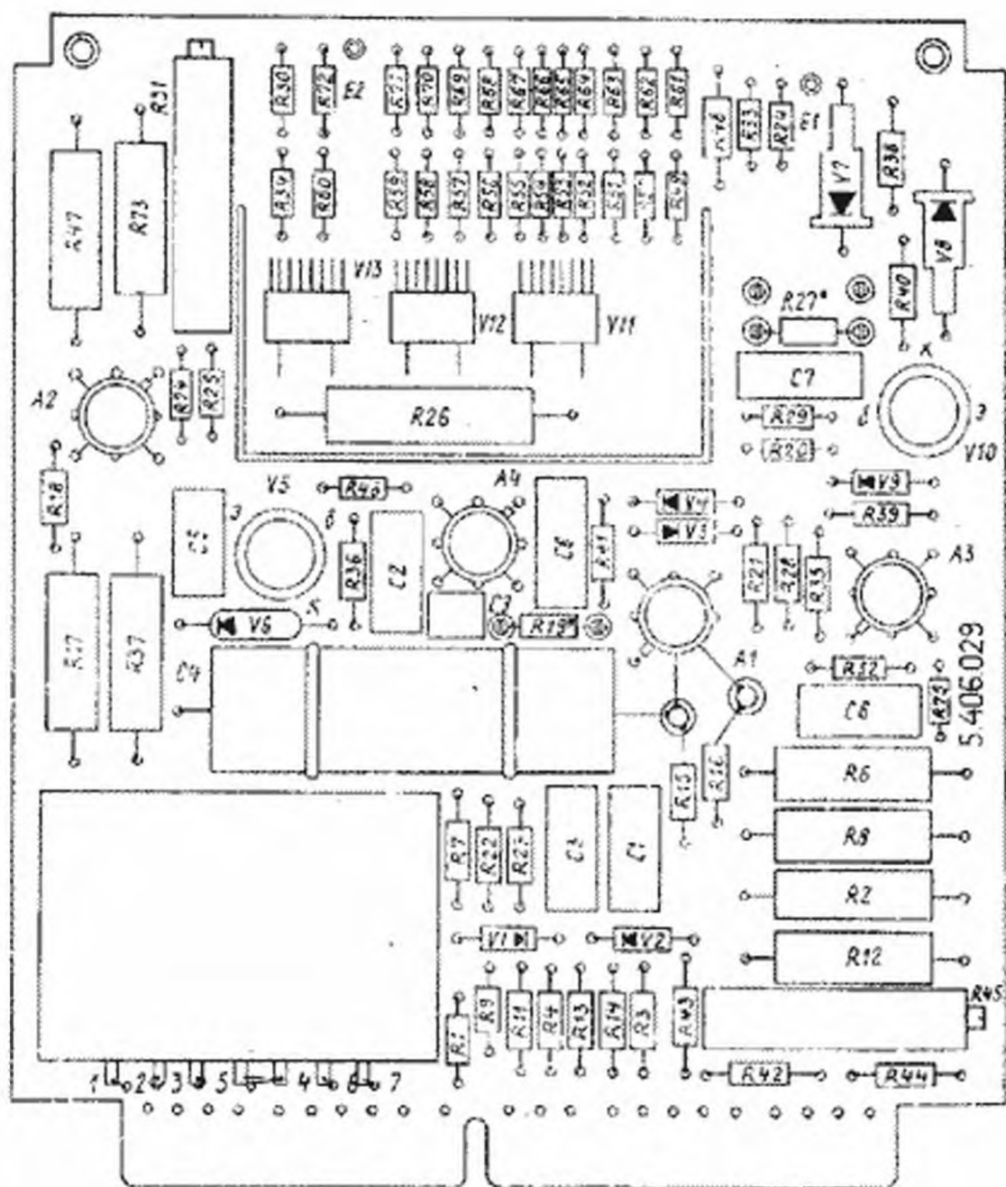
Преобразователь (пл. 5.406.029)
