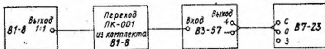
Рис. 10. Схема соединения аппаратуры при определении основной приведенной погрешности выходного напряжения прибора.
