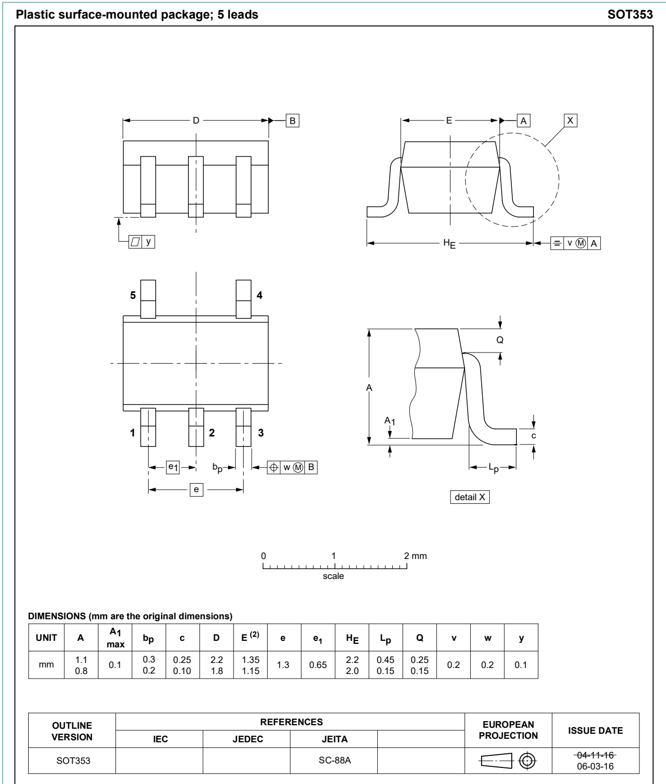
Fig. 1. Package outline TSSOP5 (SOT353)
