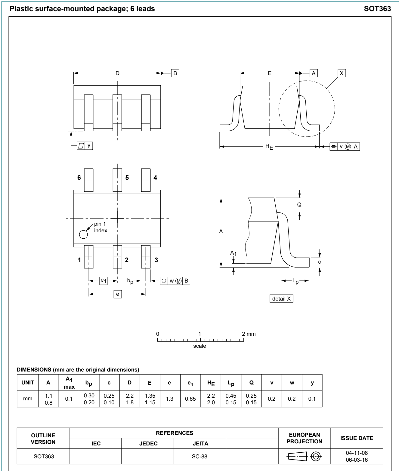
Fig. 1. Package outline TSSOP6 (SOT363)
