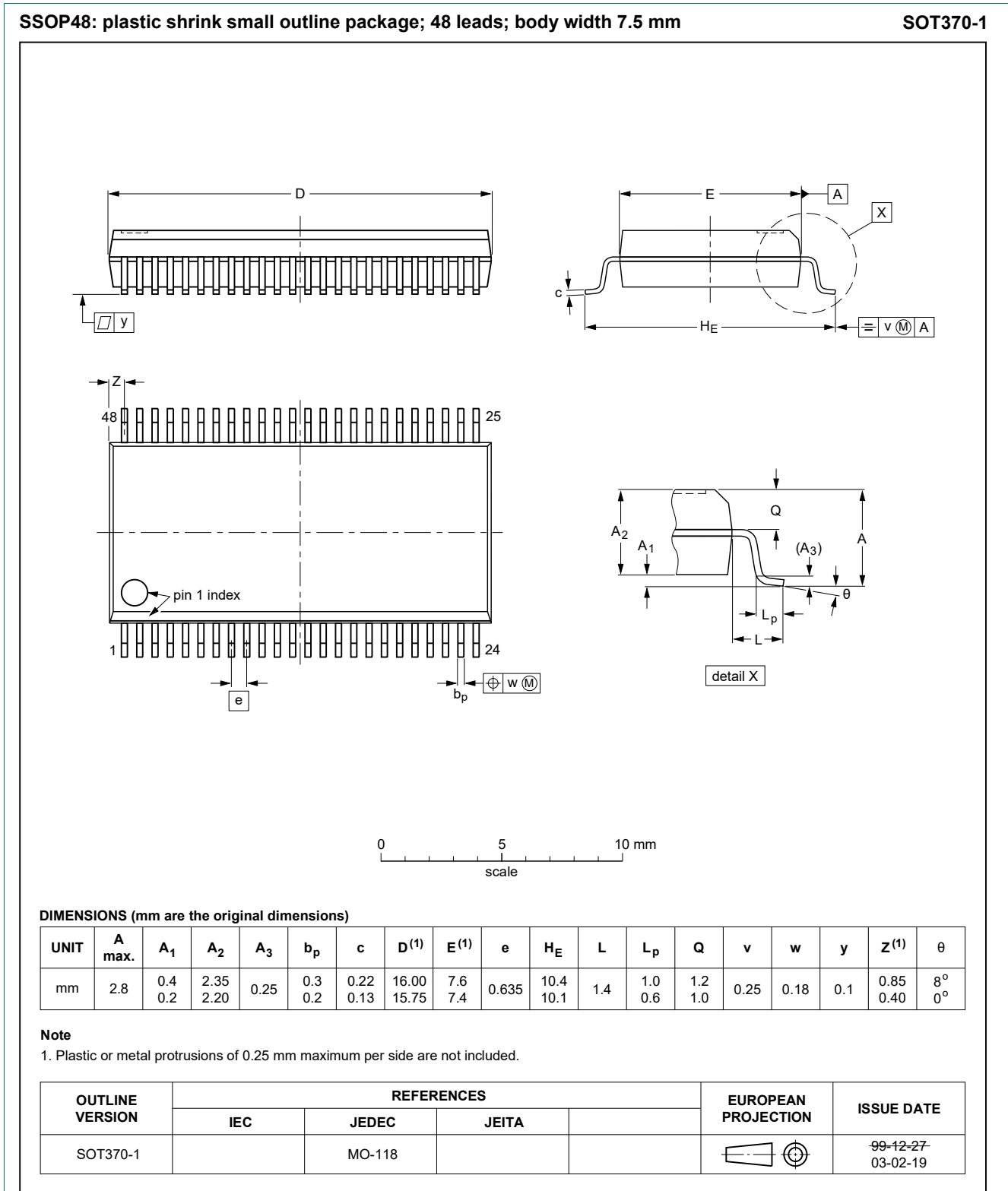
Fig. 1. Package outline SSOP48 (SOT370-1)
