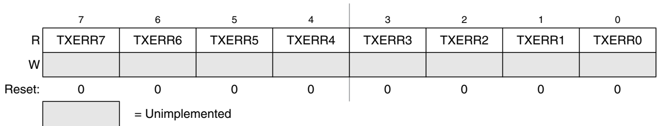
Figure 12-18. MSCAN Transmit Error Counter (CANTXERR)
