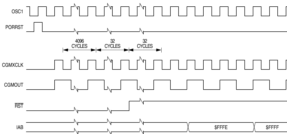
Figure 14-8. POR Recovery
