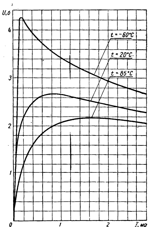
Ориентировочная вольт-амперная характеристика термистора ТПМ2/0,5А
