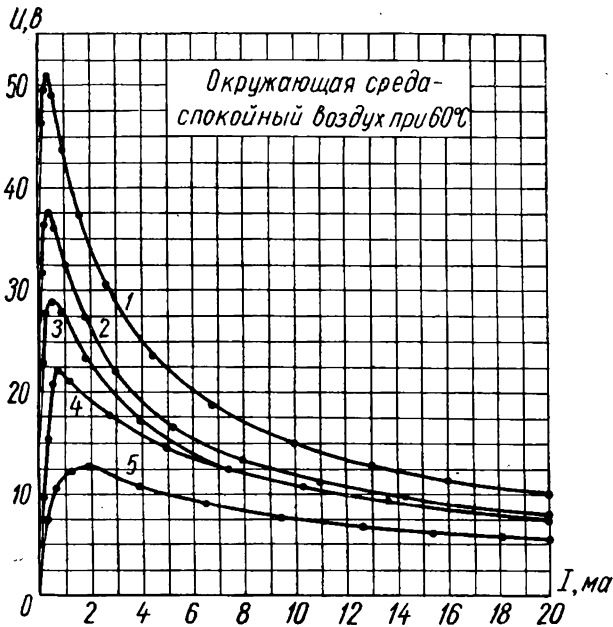
Вольт-амперные характеристики термосопротивлений КМТ-10
