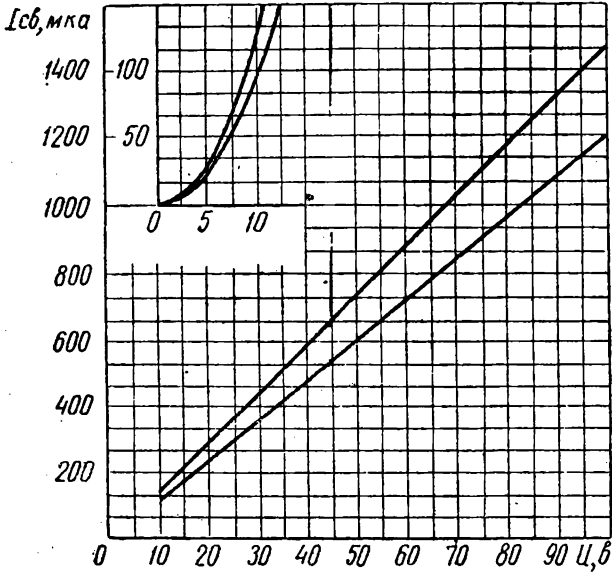
Зависимость светового тока I_{сз} от рабочего напряжения при освещенности 200 лк (вольтамперные характеристики)
