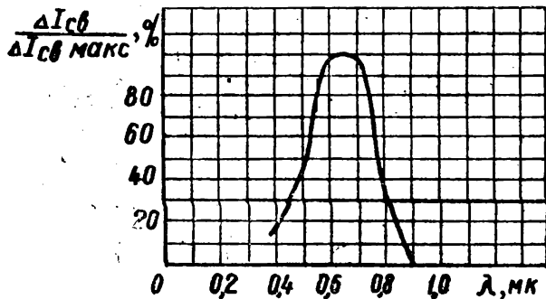
Спектральная чувствительность
