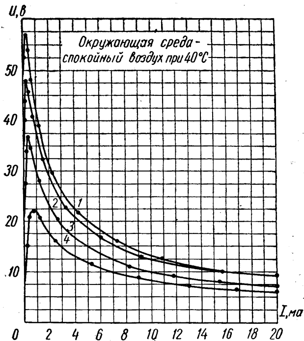
Вольт-амперные характеристики термосопротивлений KMT-11
