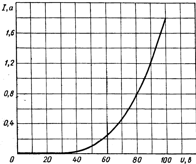
Вольт-амперная характеристика
