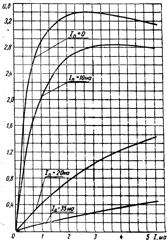
Ориентировочная вольт-амперная характеристика термистора ТКП-50 при различных токах подогревателя
