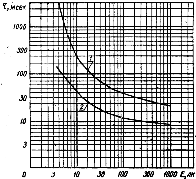
Зависимость постоянной времени \tau от освещенности E
