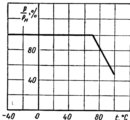
P — допускаемая мощность нагрузки, вт ; P_n — номинальная мощность рассеяния, вт .
