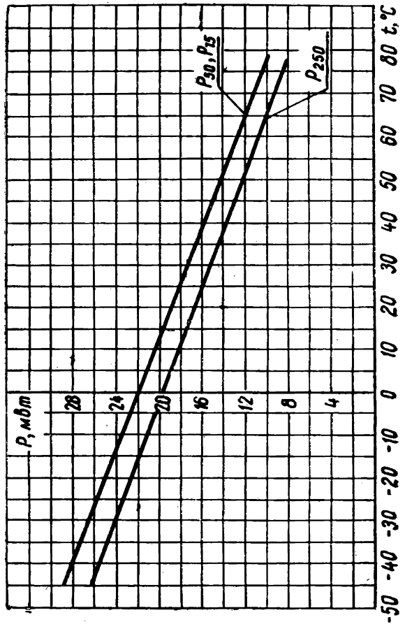
Ориентировочная зависимость рабочей мощности термистора от температуры
