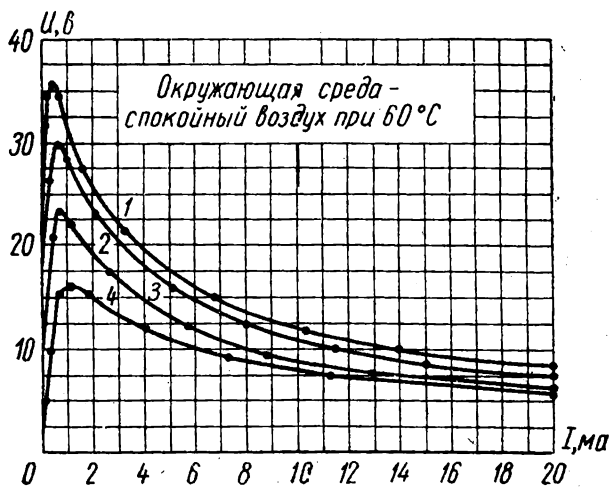
Вольт-амперные характеристики термосопротивлений KMT-11
