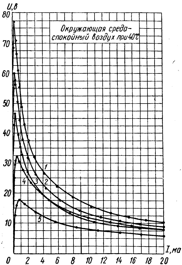
Вольт-амперные характеристики термосопротивлений KMT-10
