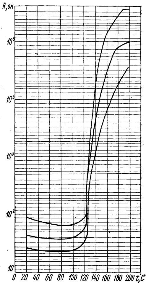
Зависимость сопротивления терморезисторов от температур окружающего воздуха
