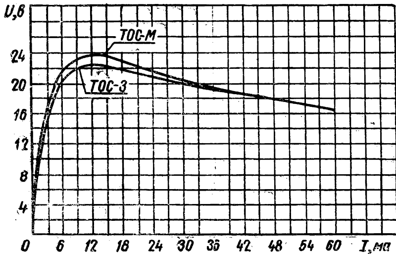
Ориентировочная вольт-амперная характеристика
