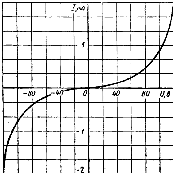
Вольт-амперная характеристика
