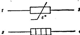
Электрическая схема
