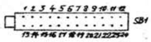
Схема нумерации выводов переключателей (вид со стороны печатного монтажа)
