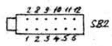
Схема нумерации выводов переключателей (вид со стороны печатного монтажа)
