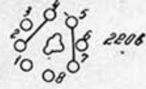
Положение переключателя П1
