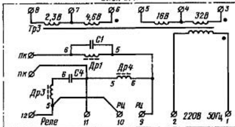
Блок БРК
