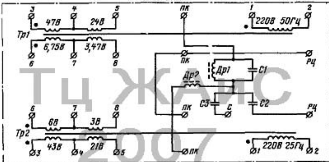
Блок БРК
