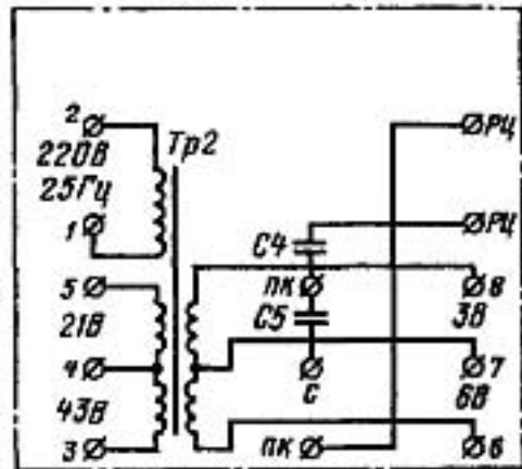
Блок БП
