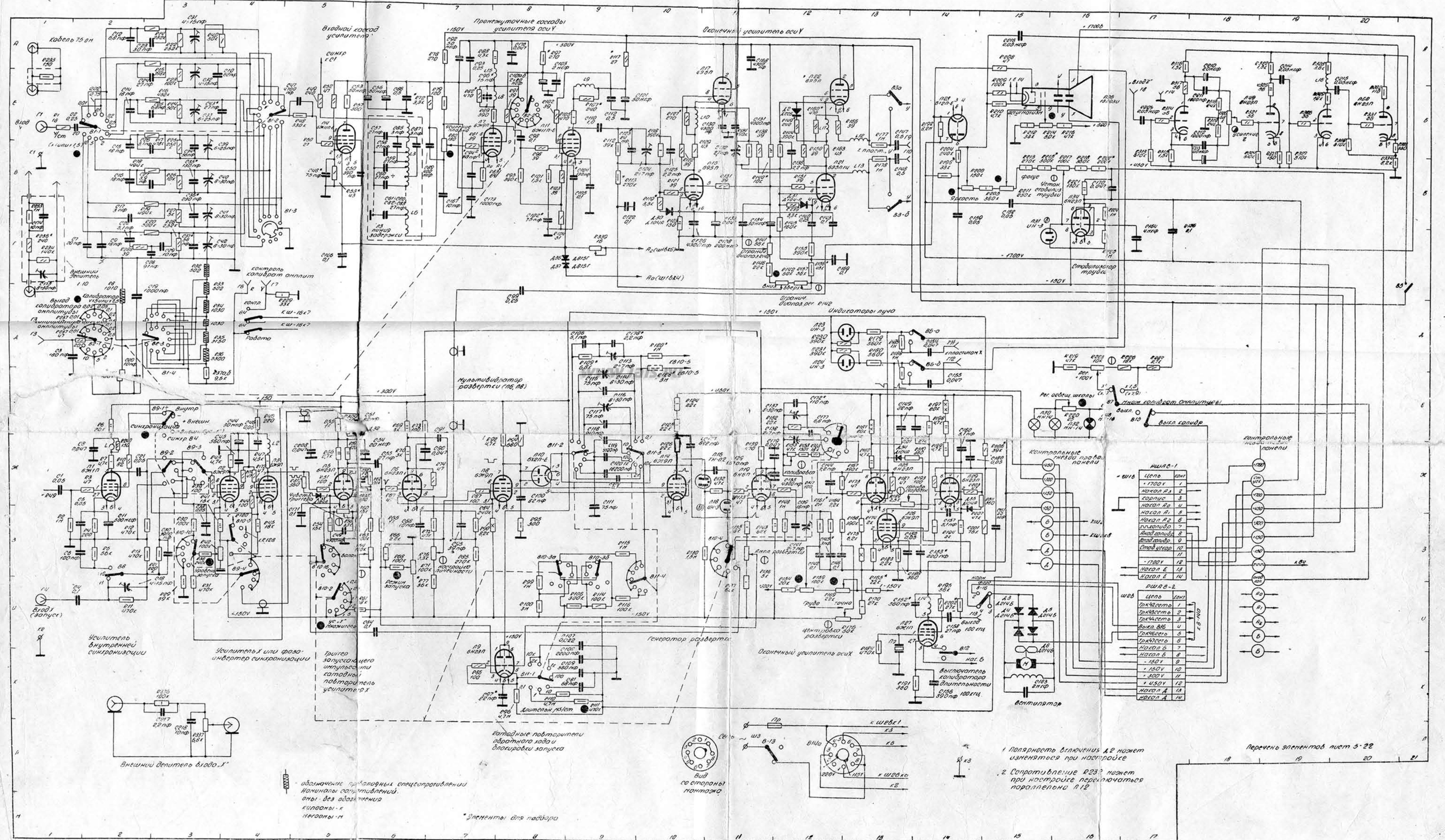
ПРИНЦИПАЛЬНАЯ ЭЛЕКТРИЧЕСКАЯ СХЕМА (Измерительного блока) ПРИБОРА С1-20
